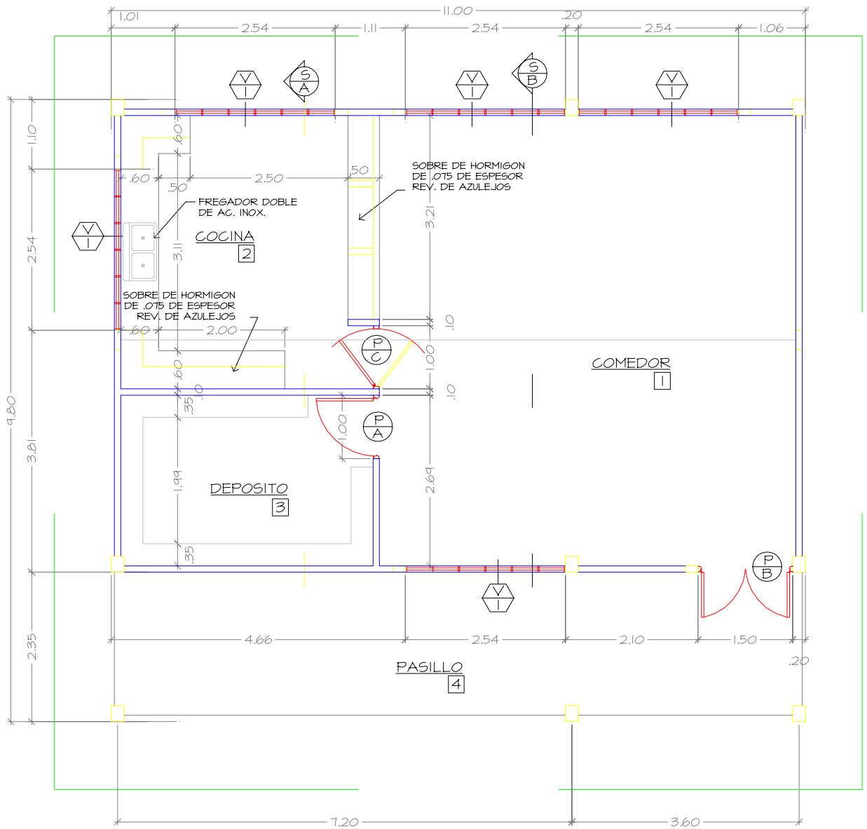
PLANTA ARQUITECTONICA TÍPICA - COCINA-COMEDOR 5/E
