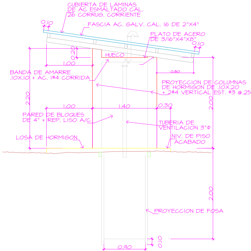
ELEVACION LATERAL DE LETRINA S/E
