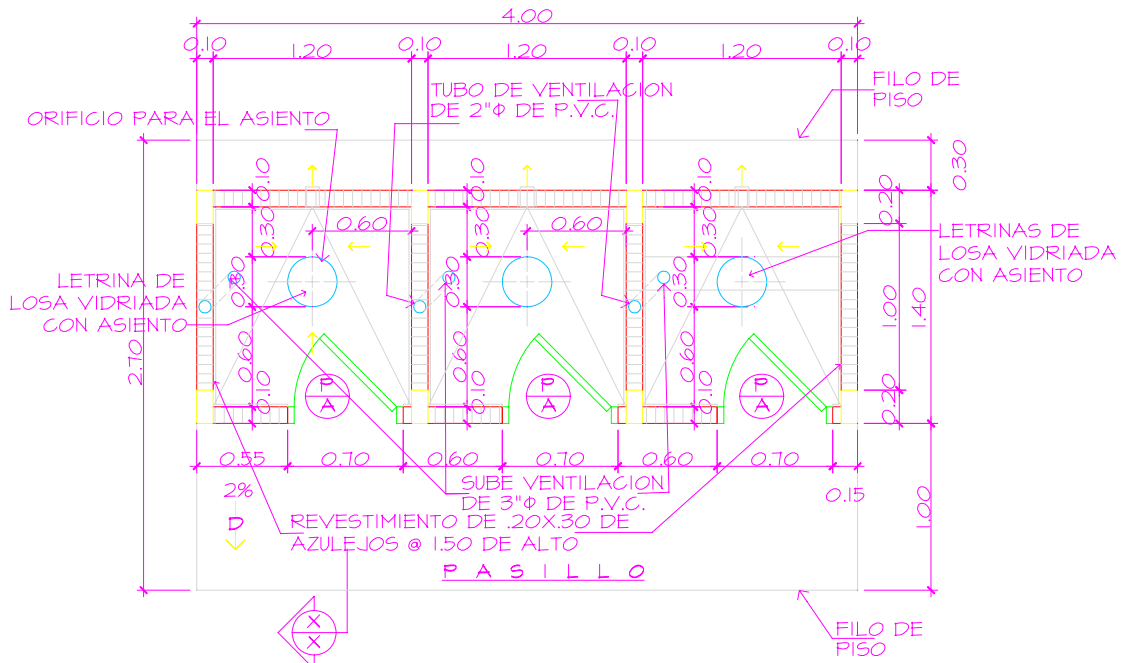
PLANTA ARQUITECTONICA DE LETRINA S/E
