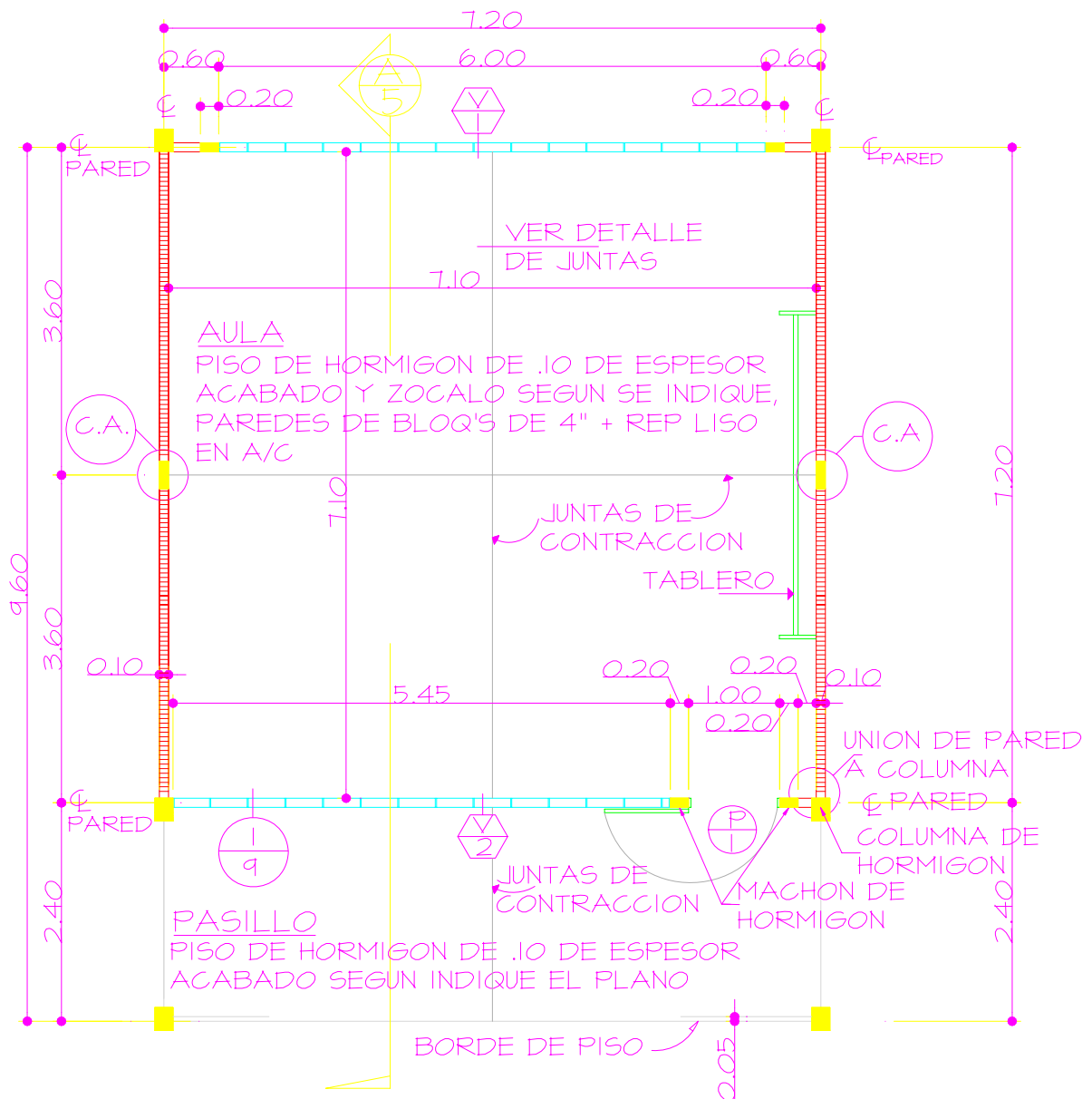
PLANTA ARQUITECTONICA UN AULA TIPICA S/E
