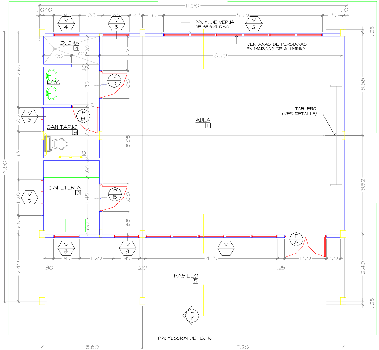
PLANTA ARQUITECTONICA TIPICA - PRE-ESCOLAR 5/E
