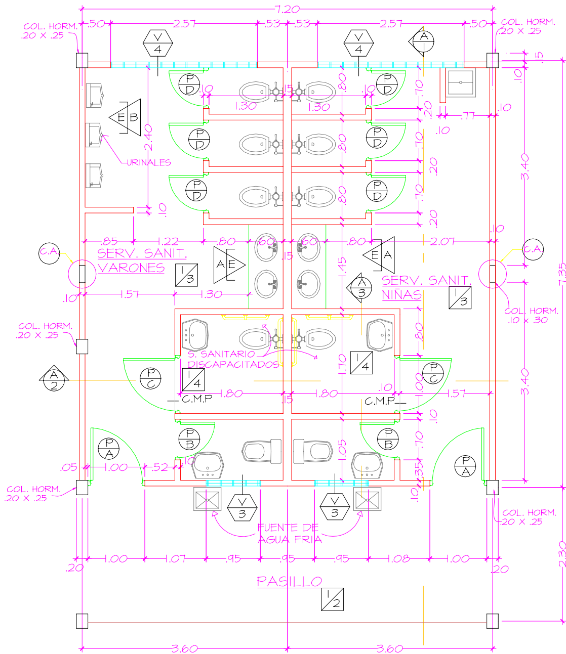
PLANTA ARQUITECTONICA TIPICA SERVICIO SANITARIO
